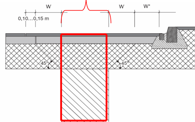
,theoretische' Grabenbreite
