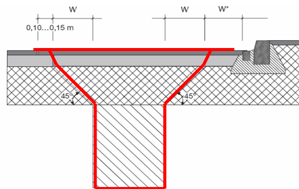
Aufgrabung
